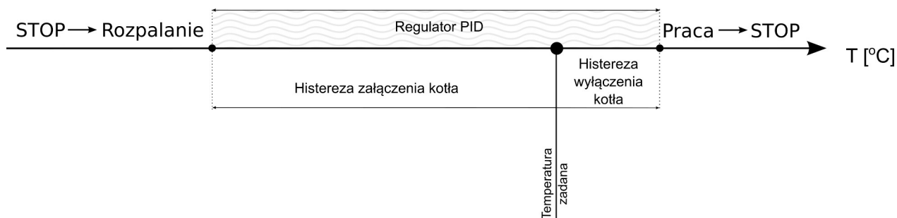
Ilustracja 19: Schemat przełączania się algorytmu spalania między mocami dla regulatora procesu spalania PID
