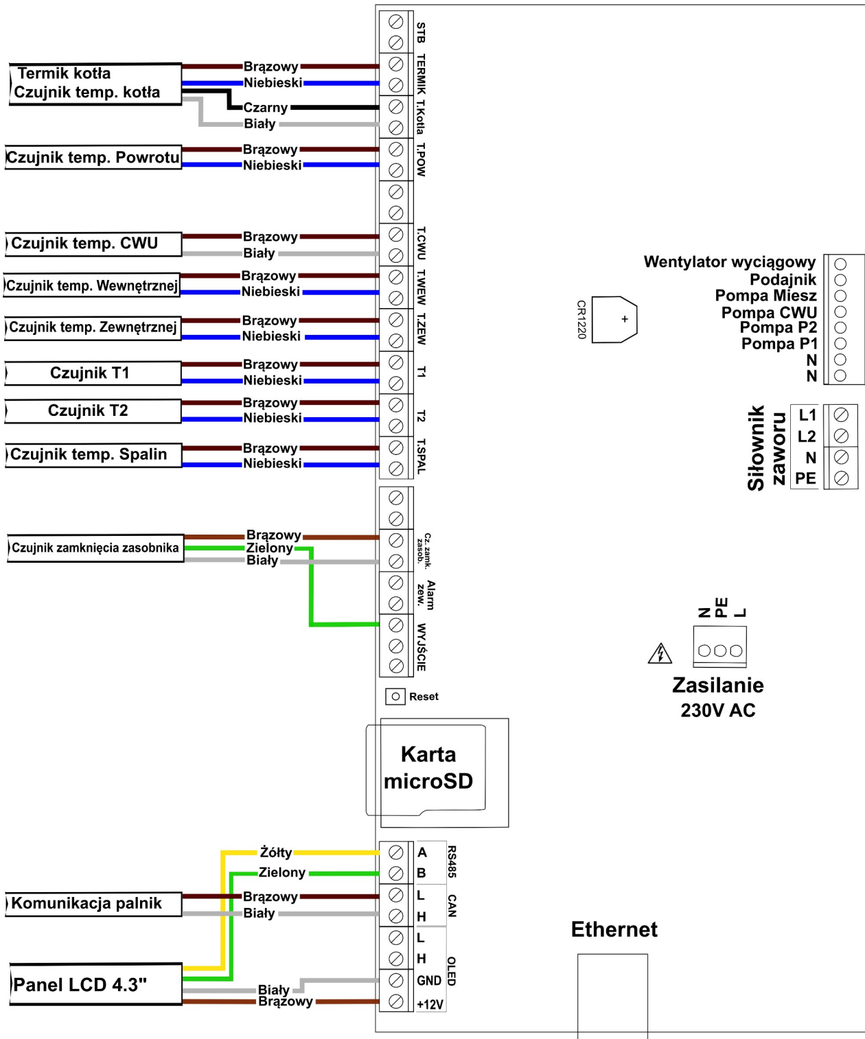
Ilustracja 3: Listwa zaciskowa do podłączenia czujników
