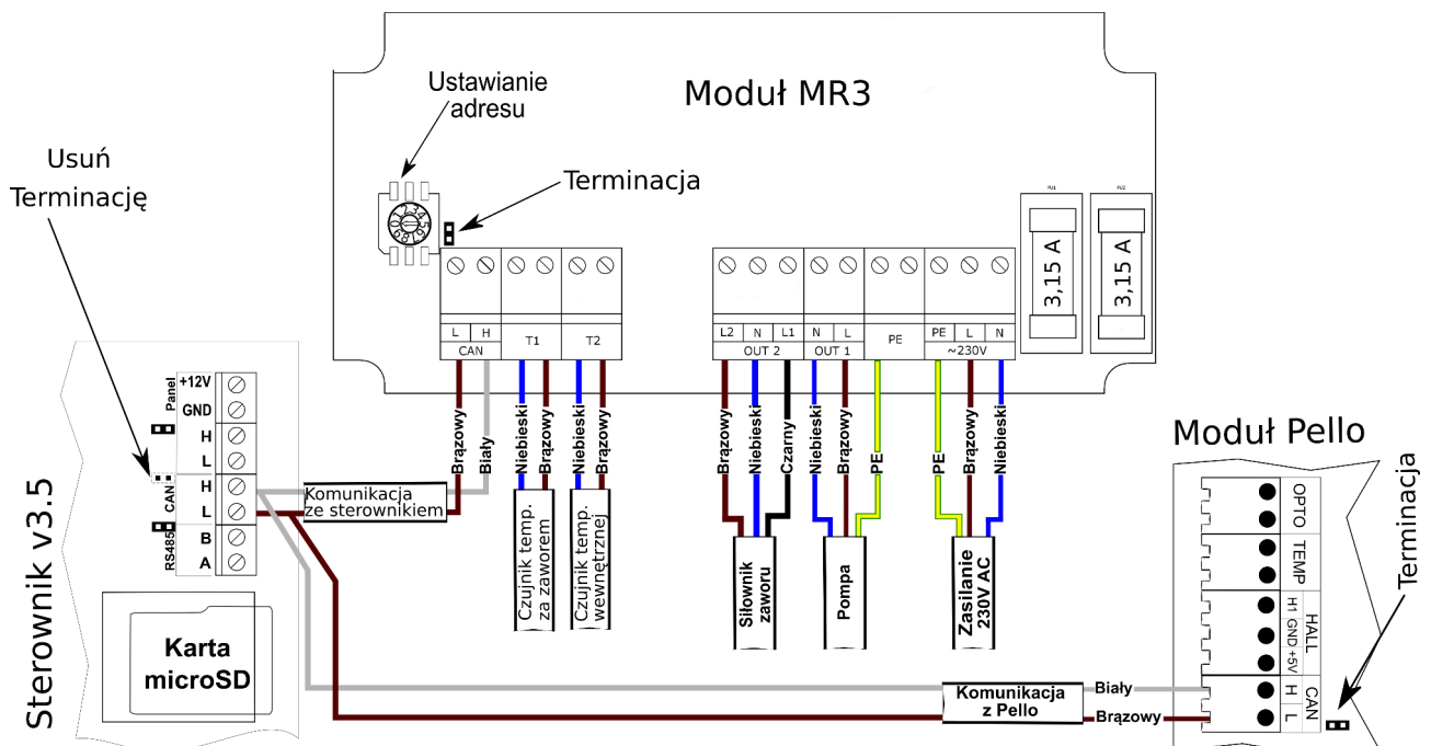
Ilustracja 7: Schemat podłączenia modułu rozszerzeń MR3.
