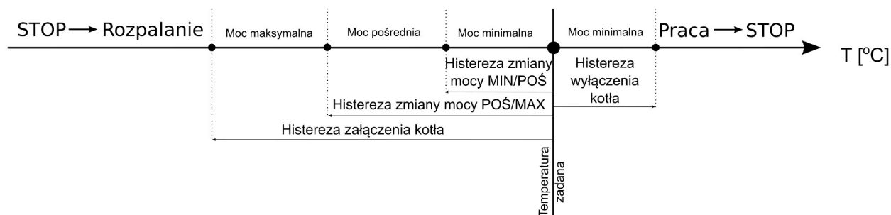
Ilustracja 18: Schemat przełączania się algorytmu spalania między mocami dla regulatora procesu spalania Auto
