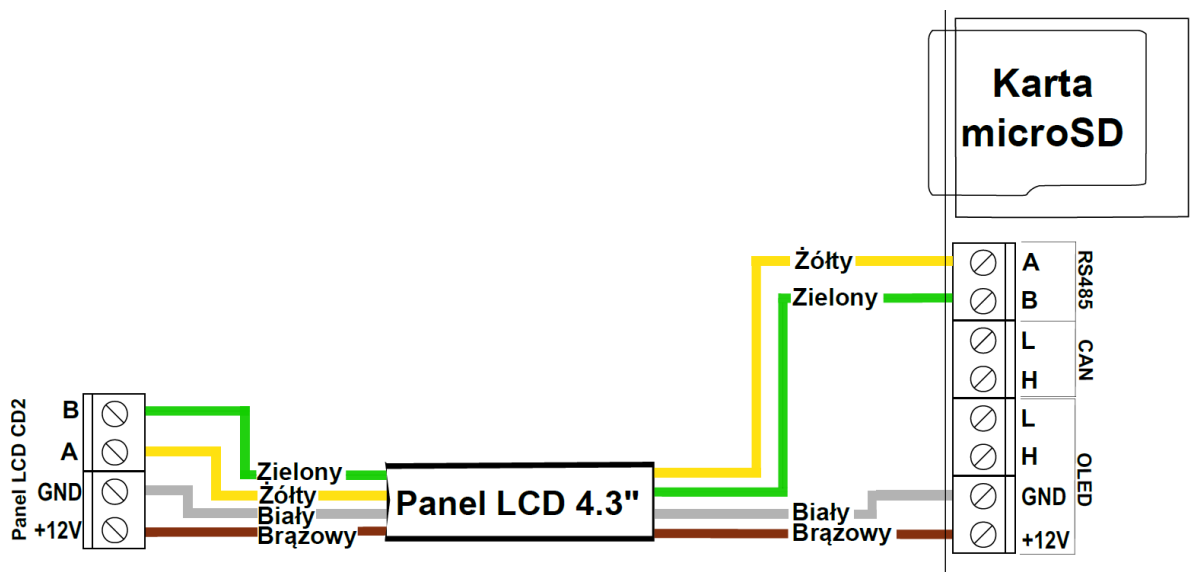
Ilustracja 1: Wyprowadzenia wtyczki przewodu do panelu CD2 4.3"
