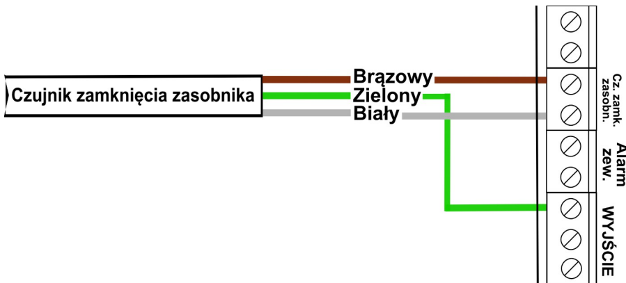
Ilustracja 6: Podłączenie czujnika zamknięcia zasobnika
